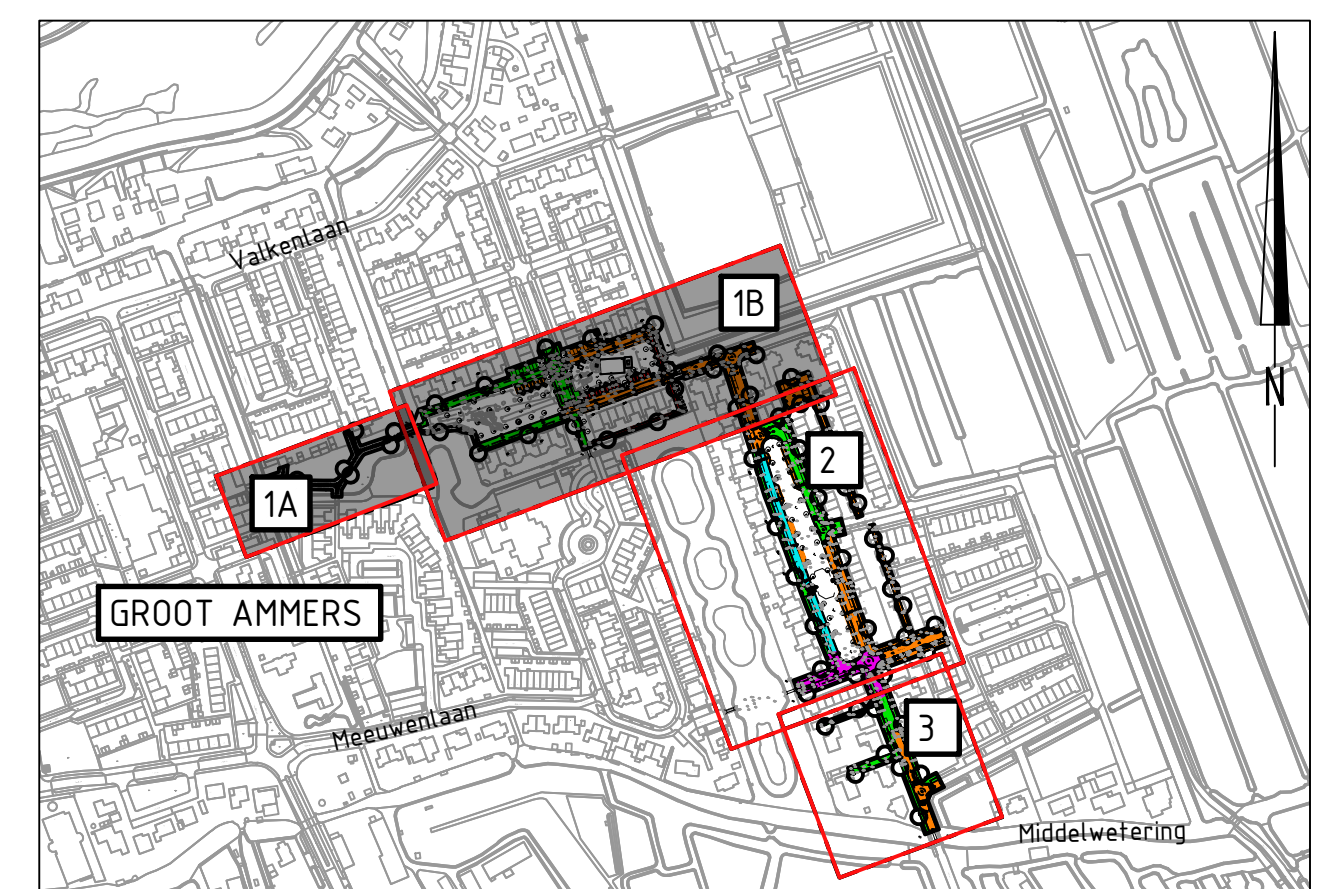
OVERZICHTSTEKENING Schaal 1:5000
