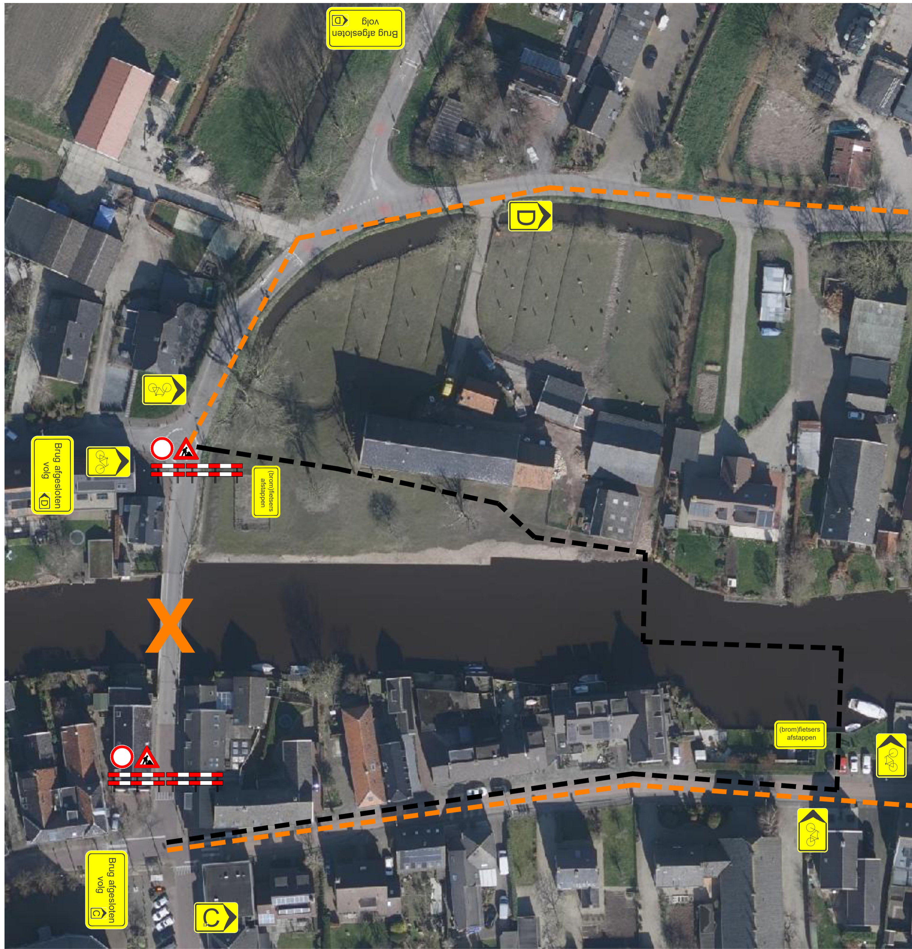
Detail brugstraat Schaal: 1:50
