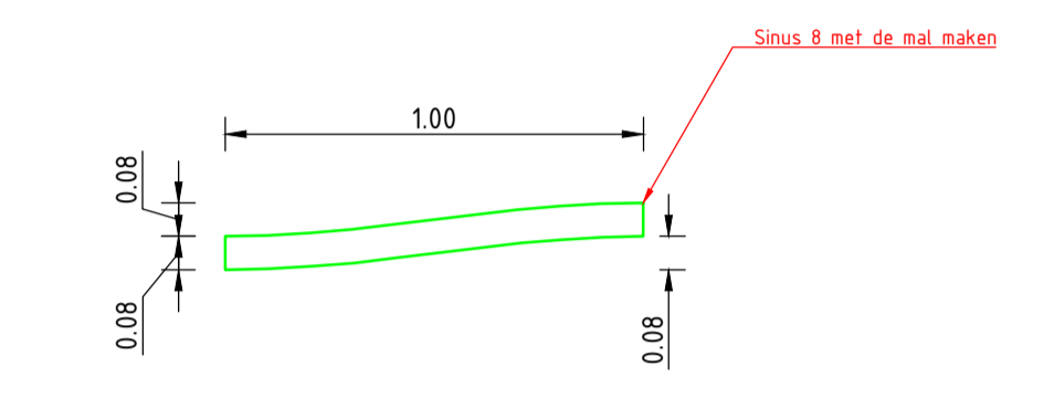
Doorsnede verkeersdrempel Sinus 8 Schaal 1:20
