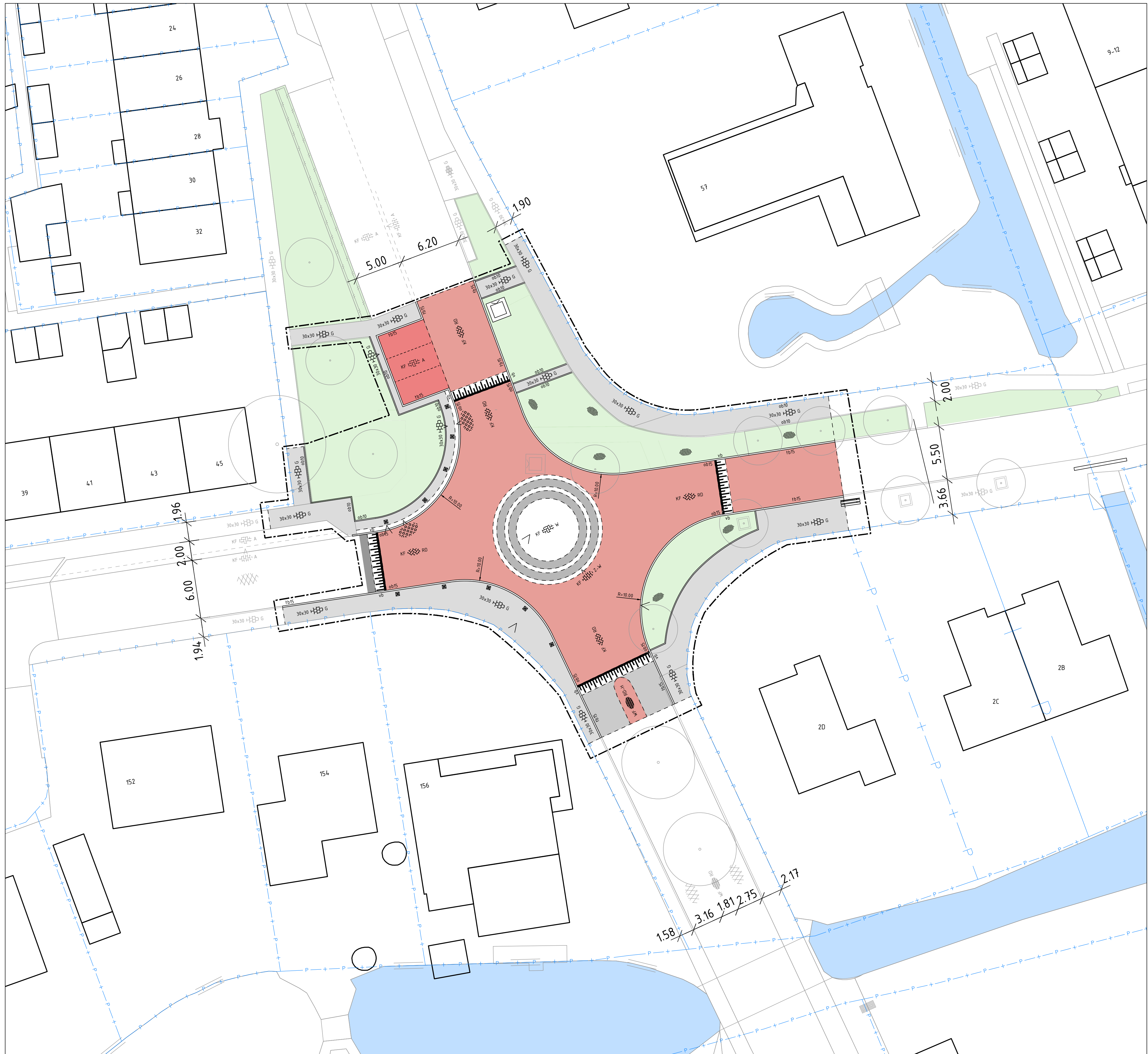
OVERZICHT SCHAAL 1:200
