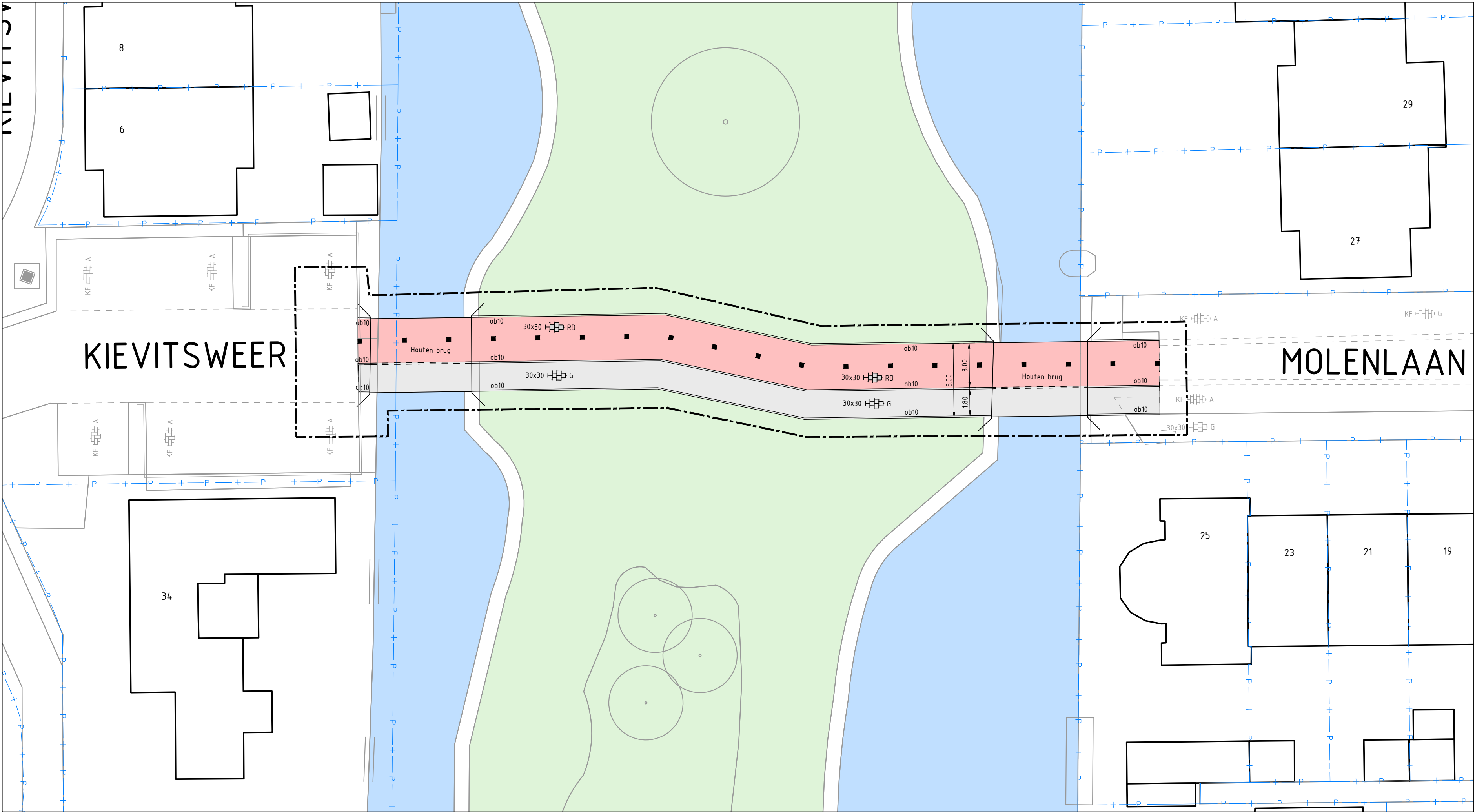
OVERZICHT SCHAAL 1:200
